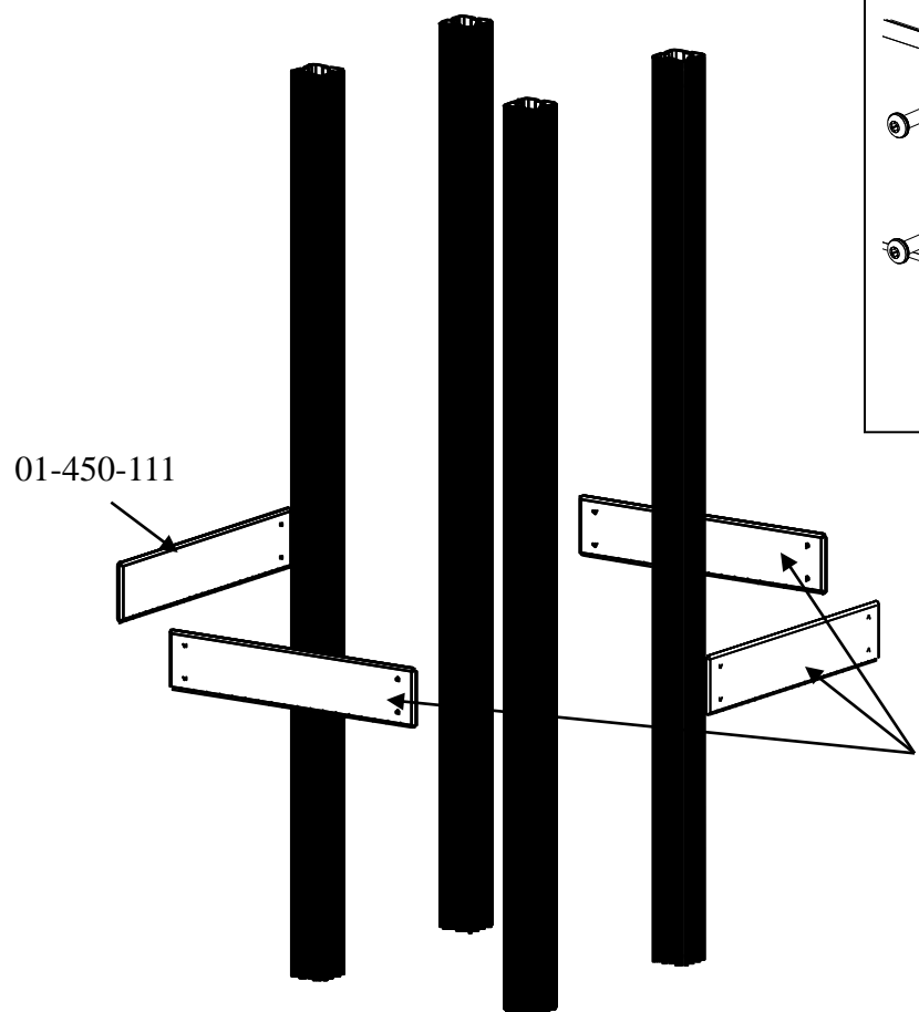
01-450-111
