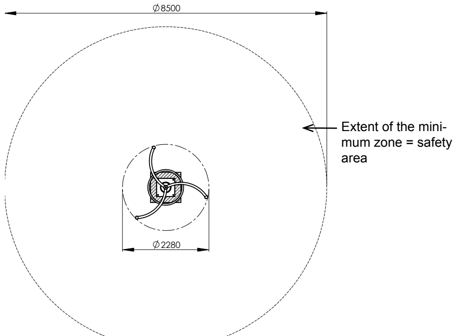
Diagram 3: Top view „ventus“
